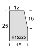
Hochbordprofil im Schrankenbereich
